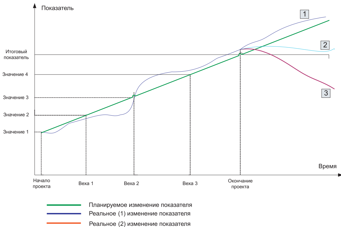
Рисунок 21. Жизнеспособность проекта
